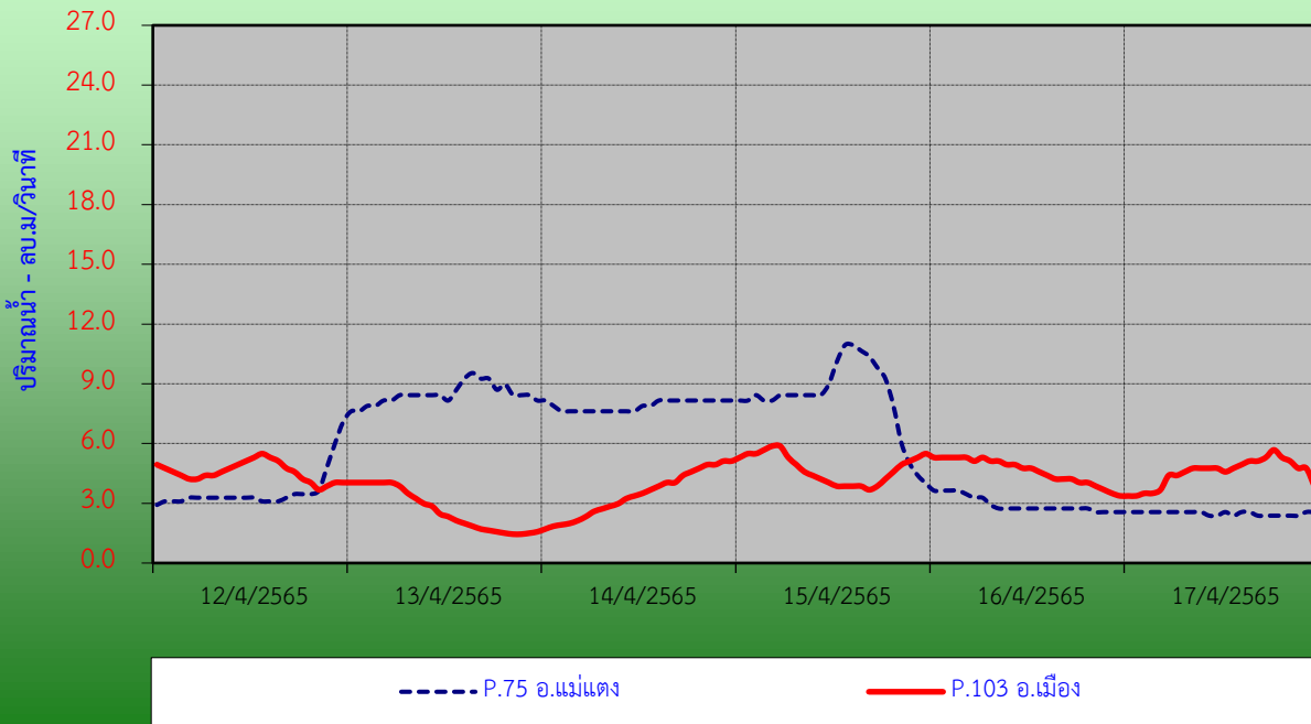
กราฟแสดงปริมาณน้ำปิ้งรายชั่วโมงรอบวันที่ 15/2565 ที่สถานีแม่ น้ำปิ้ง (P.75) บ้านซ้อแล อ.แม่แตง และที่สถานีแม่ น้ำปิ้ง(P.103) บ้านป่าซ่อยใต้ อ.เมือง จ.เชียงใหม่
